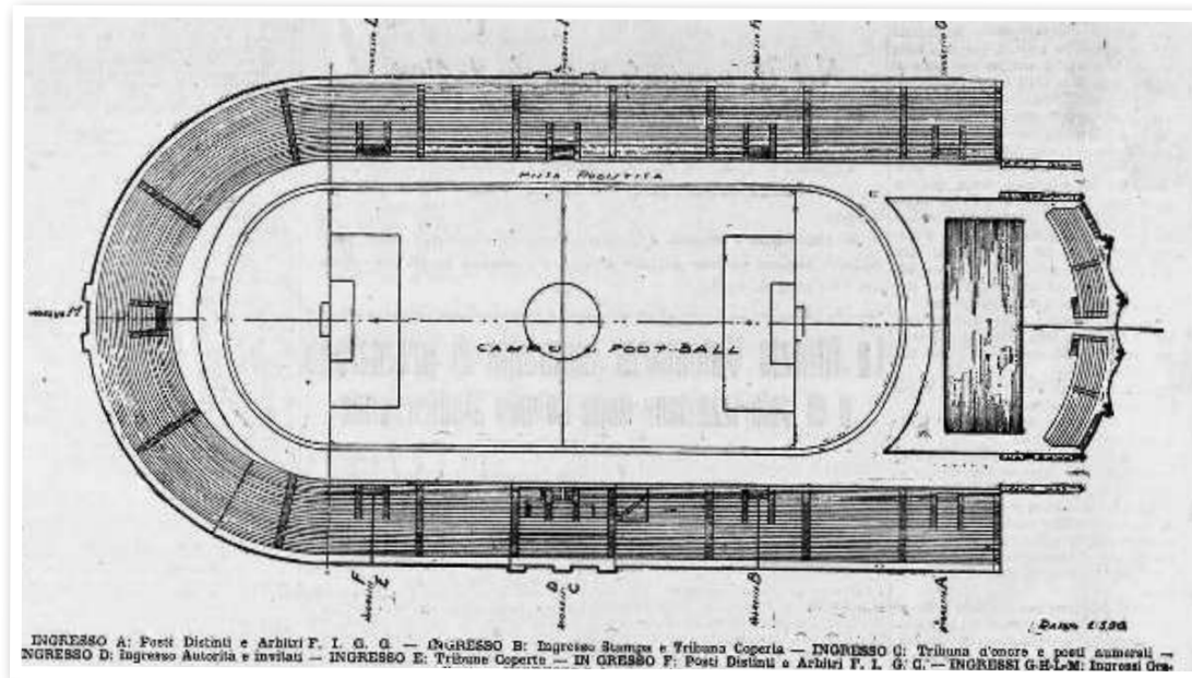
La pianta dello Stadio del PNF
