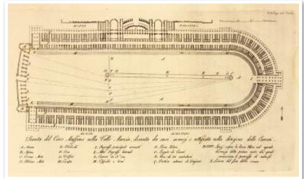
Pianta del Circo Massimo
