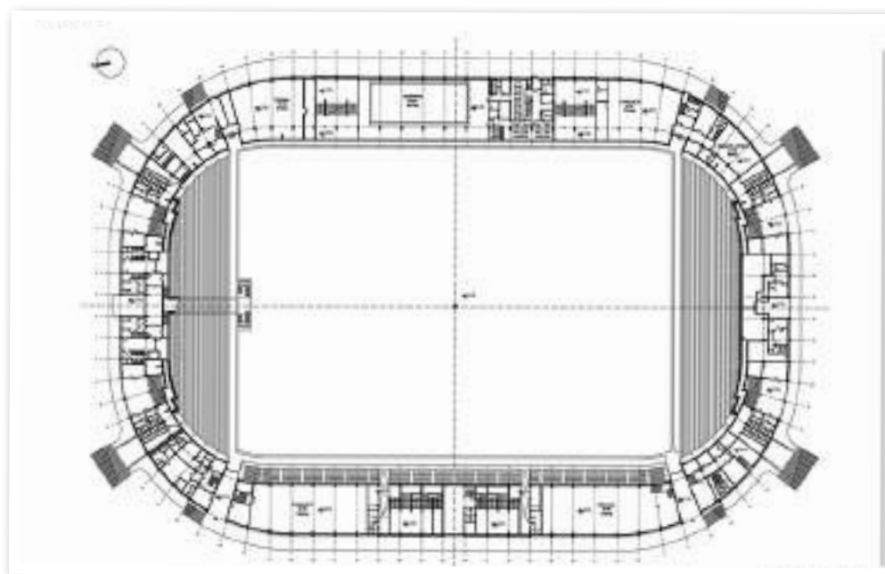
Pianta dello Stadio Flaminio
